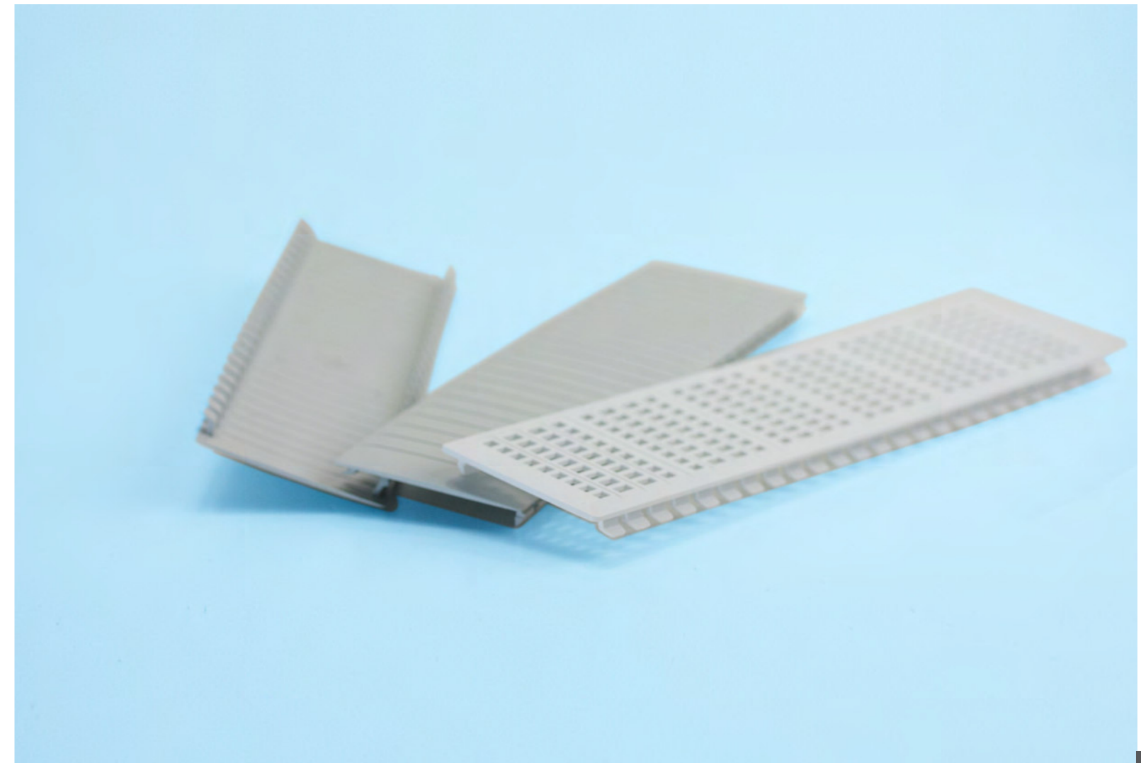
Blindabdeckungen | Blanking plates | Obturateurs
